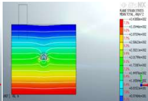
Fig 7 : Stress
