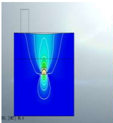
Fig 3 : Total displacement.
