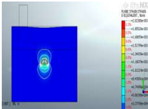
Fig 6 : Strain equivalent.
